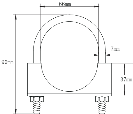
U型卡寸图
